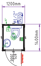
Kontener WC 5'
